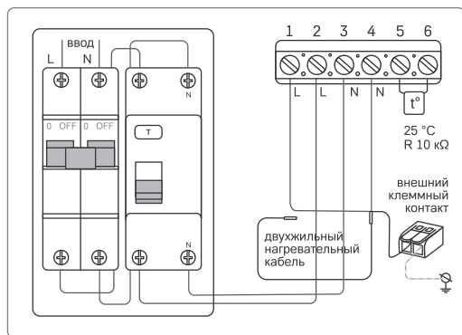
Схема 1. Пример подключения двухжильного нагревательного кабеля к терморегулятору Welrok. Схема соответствует моделям терморегулятора: Welrok oz, Welrok az, Welrok pro, Welrok lis, Welrok st.
