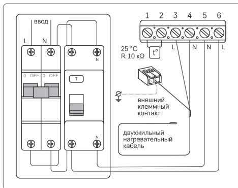
Схема 2. Пример подключения двухжильного нагревательного кабеля к терморегулятору Welrok. Схема соответствует моделям терморегулятора: Welrok rtp, Welrok mex.
